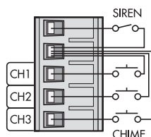
10 Anschluss Gongtaster/Sirenenwechsler
