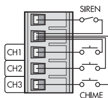
10) Podłączanie przycisków monostabilnych gongu oraz włącznika syreny
